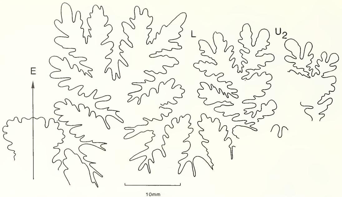
TEXT-FIG. 5. Suture of Brahmaïtes (Brahmaïtes) brahma (Forbes, 1846), BMNH C10535.
